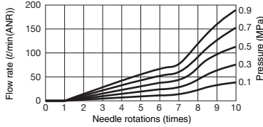
PJNMU 8 (PJNMU 5/16) Control flow
