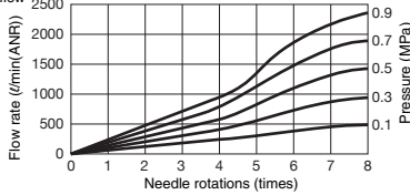
PJNMU 1/2 PJNMU 12 Control flow
