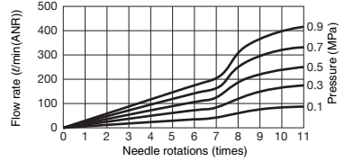
PJNMU 3/8 PJNMU 10 Control flow
