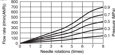
PJNMU 1/2 PJNMU 12 Control flow
