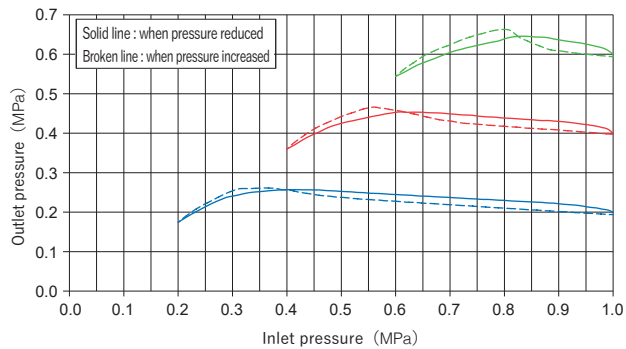
RVCP3/16-N2U
