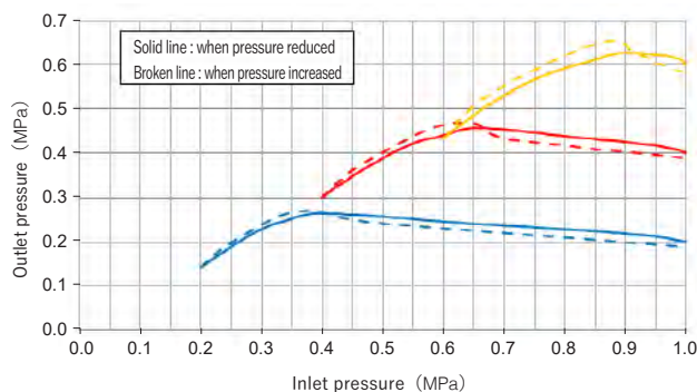
RVCP3/16-N2U
