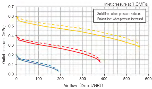
RVCP1/4-N2U, RVCMP1/4-N2U
