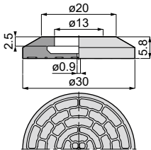
VP30F Weight : 3.5g[5.1g]
