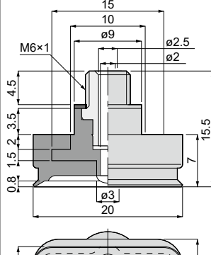
VP5×20E[5]-M6[9] Weight : 2.4g[2.8g]
