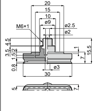
VP5×30E[5]-M6[9] Weight : 2.8g[3.4g]
