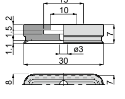
VP8×30E [5] Weight : 1.2g[1.9g]
