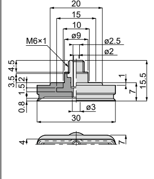
VP4×30E[5]-M6[9] Weight : 2.8g[3.5g]
