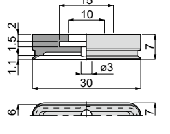
VP6×30E [5] Weight : 1.2g[1.9g]
