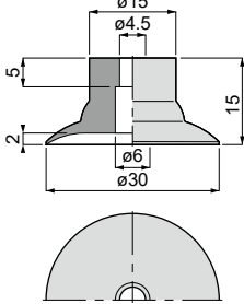
VP30L [5]
