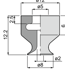
VP20L [5]
