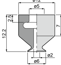
VP15L [5]
