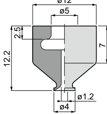
VP10L [5]
