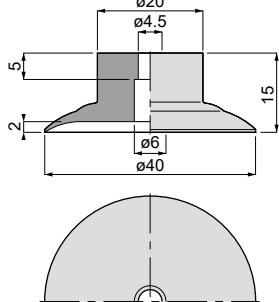
VP40L [5]
