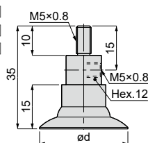
VPHE20L [5]-M5[9]
