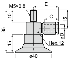
VPHE40L [5][6][9]
