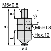
VPHE10L [5]-M5[9]
