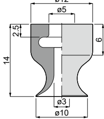
VP10L [5]
