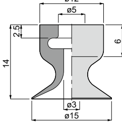
VP15L [5]
