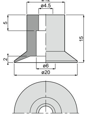
VP20L [5]
